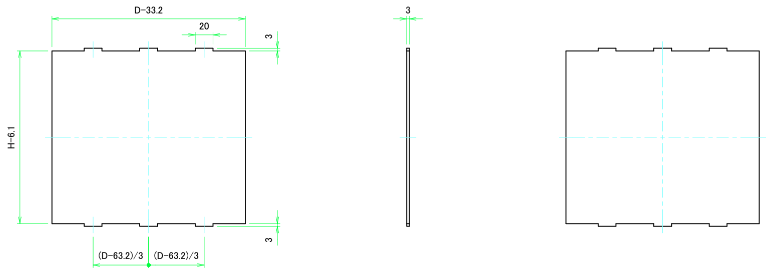
Dパネル1表面 / D Panel 1 Frontside
