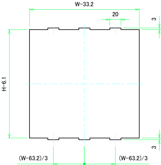
Wパネル1表面 / W Panel 1 Frontside
