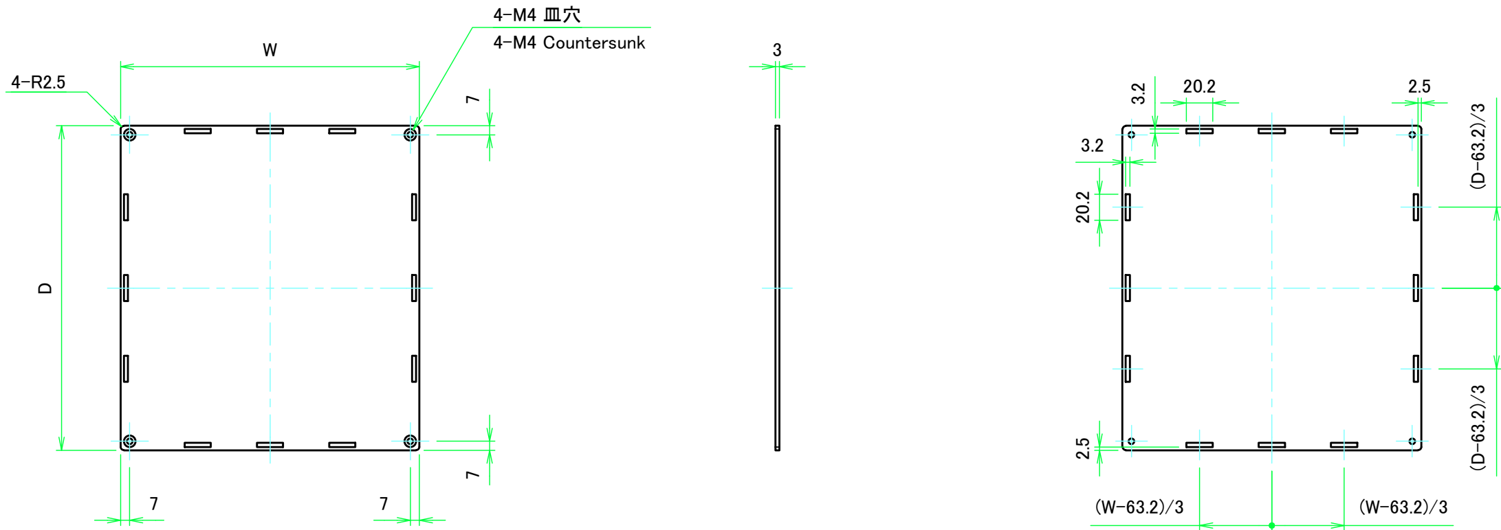
上カバー表面 / Top cover Frontside
